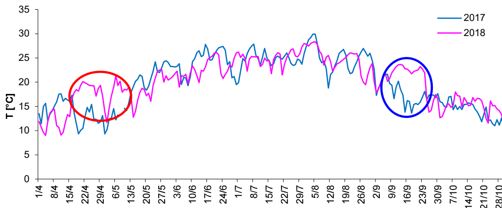
Figura 3. Confronto tra le temperature medie giornaliere 2017 e 2018 nel periodo aprile-ottobre (media tra i dati delle stazioni di Nizza Monferrato, Casale Monferrato, Alba e Cerano). Nelle ellissi sono evidenziati i periodi significativamente più caldi registrati nel 2018
